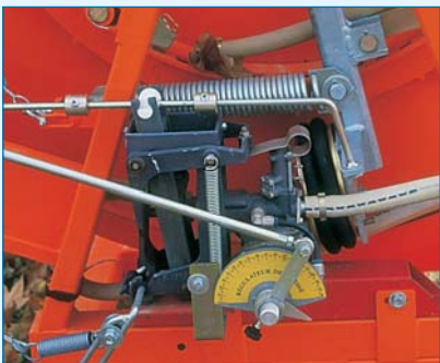
Moteur hydrobasculeur
